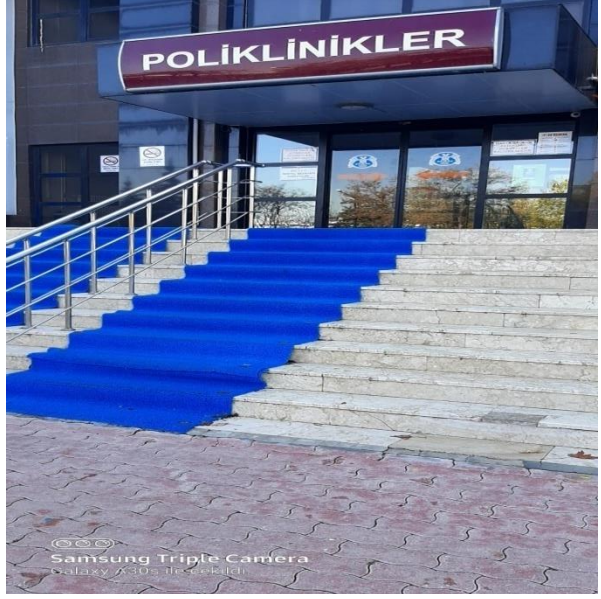
Şekil TS.7.1.7/2 Korkuluklar ve kaydırmaz halı
